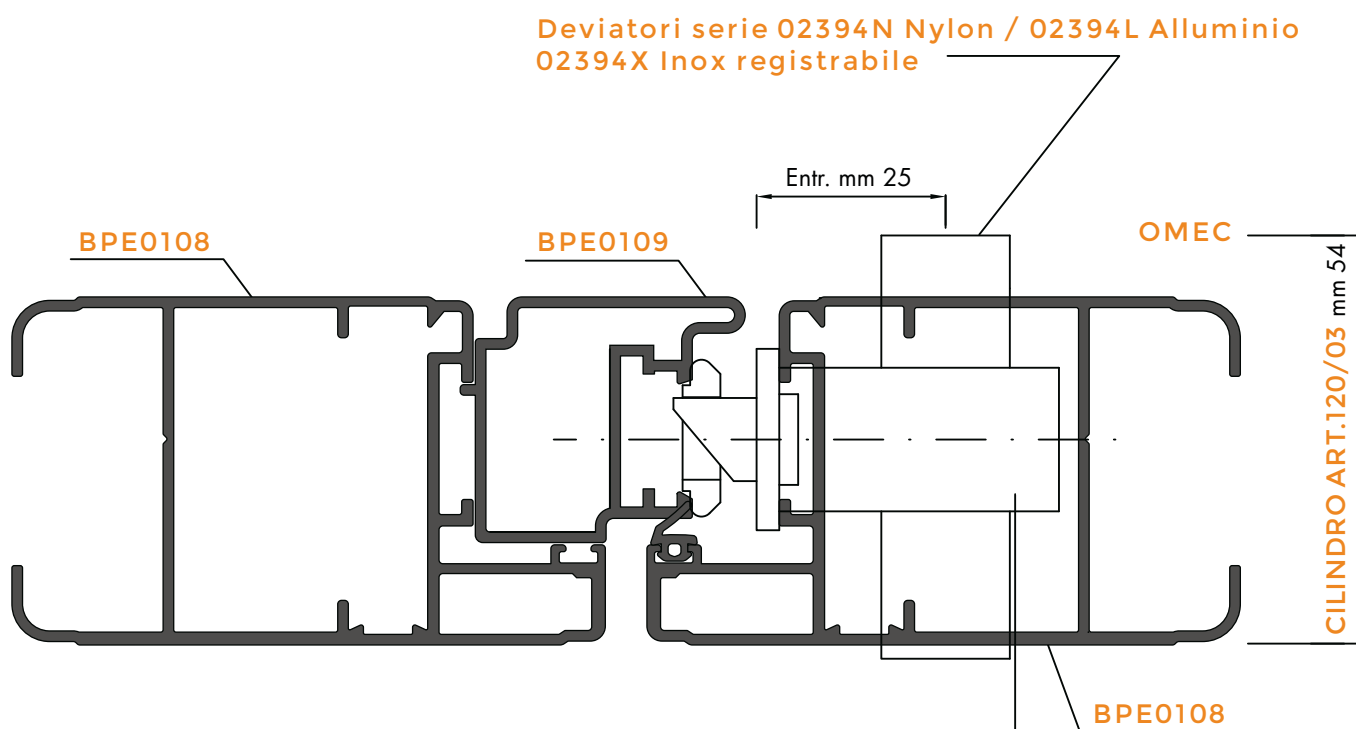
Serrature multipunto piatte serie 1560-1660
