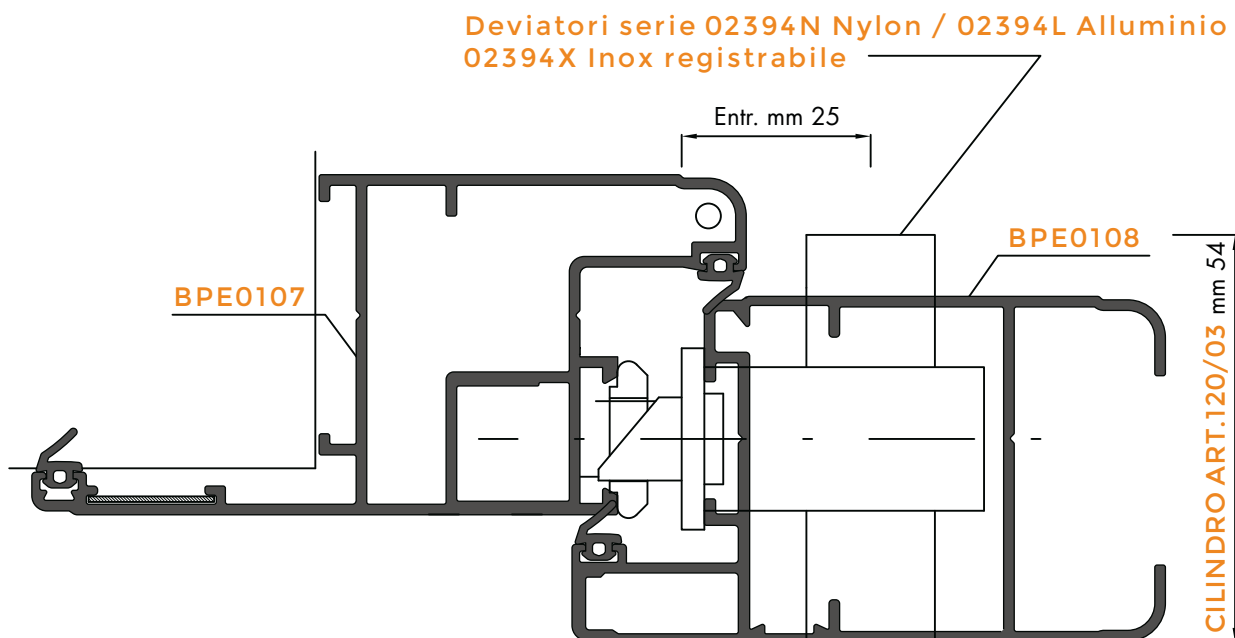
Contropiastre serrature serie 02396N Nylon 02396L Alluminio / 02396X Inox registrabile
